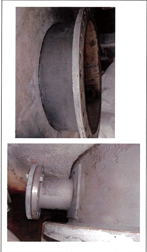
2.素地調整後状況(1種ケレン:サンドブラスト)
