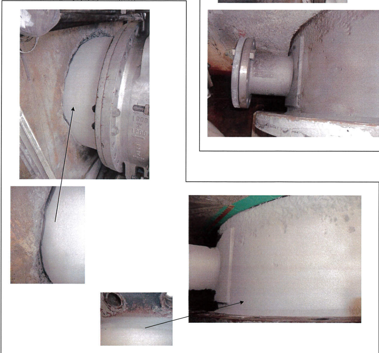
3.アーク溶射施工後状況(アルミ溶射)
